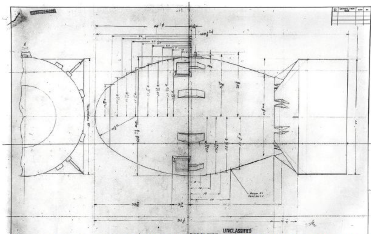
שרטוט של פצצת האטום שהוטלה על נגסאקי ב-1946. עקבות האחים נעלמו בשנות ה-50 צילום: המעבדה הלאומית לוס אלמוס/ניו יורק טיימס
