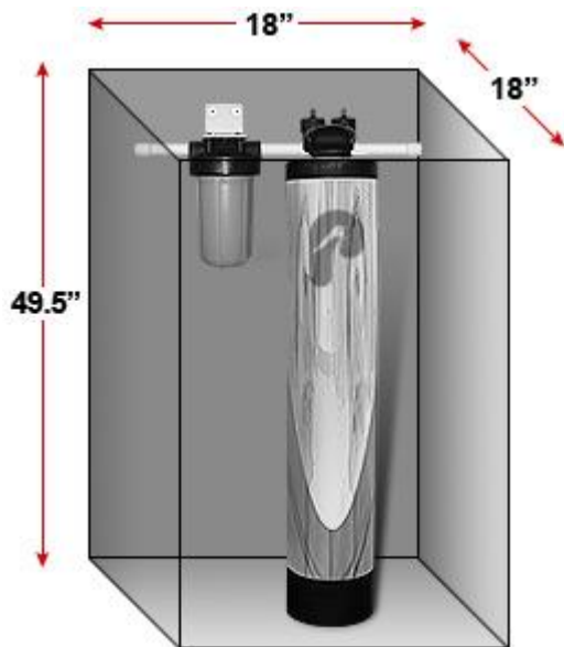
SYSTEM DIMENSIONS - NS3
