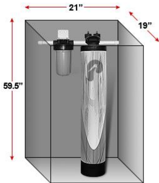
SYSTEM DIMENSIONS - NS6
