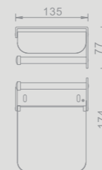
801655 מתקן לנייר טואלט
