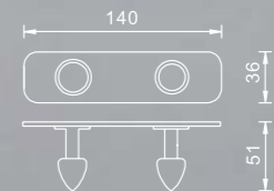
801629 קולב מגבות 2 ווים מ"מ 140x36x51
