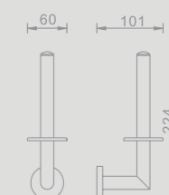
801659 מתקן לנייר טואלט הרבי
