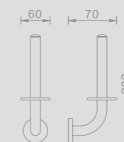
801658 מתקן לנייר טואלט הרבי
