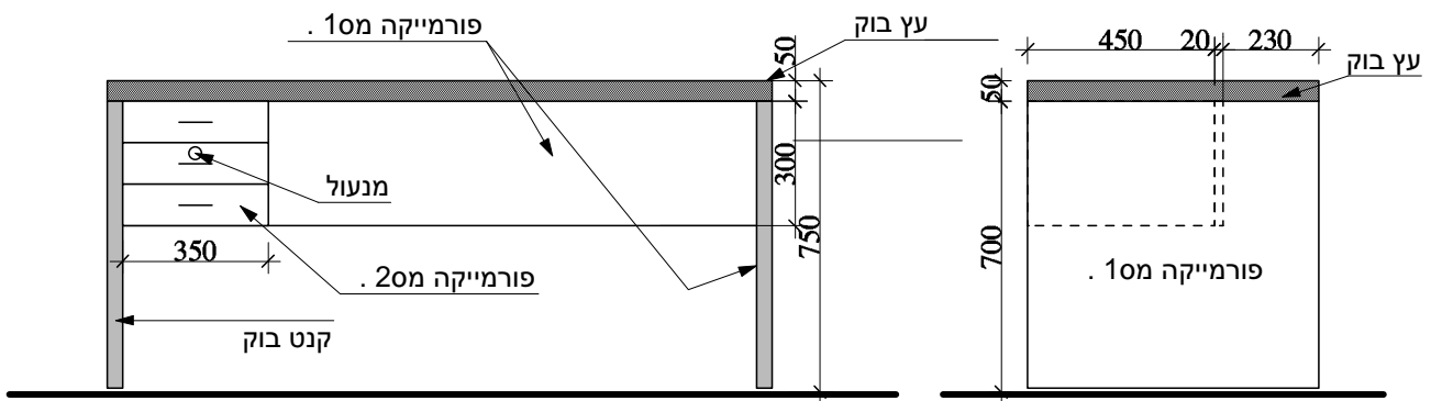
1:20 חזית
