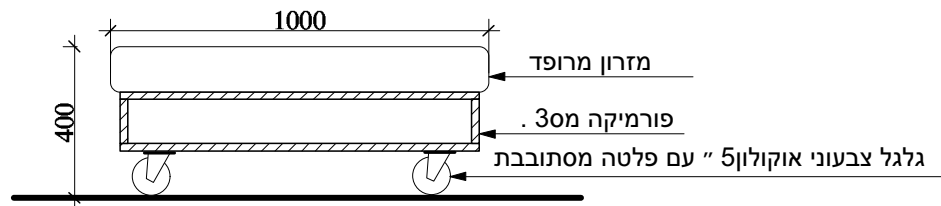
חתך 1:20
