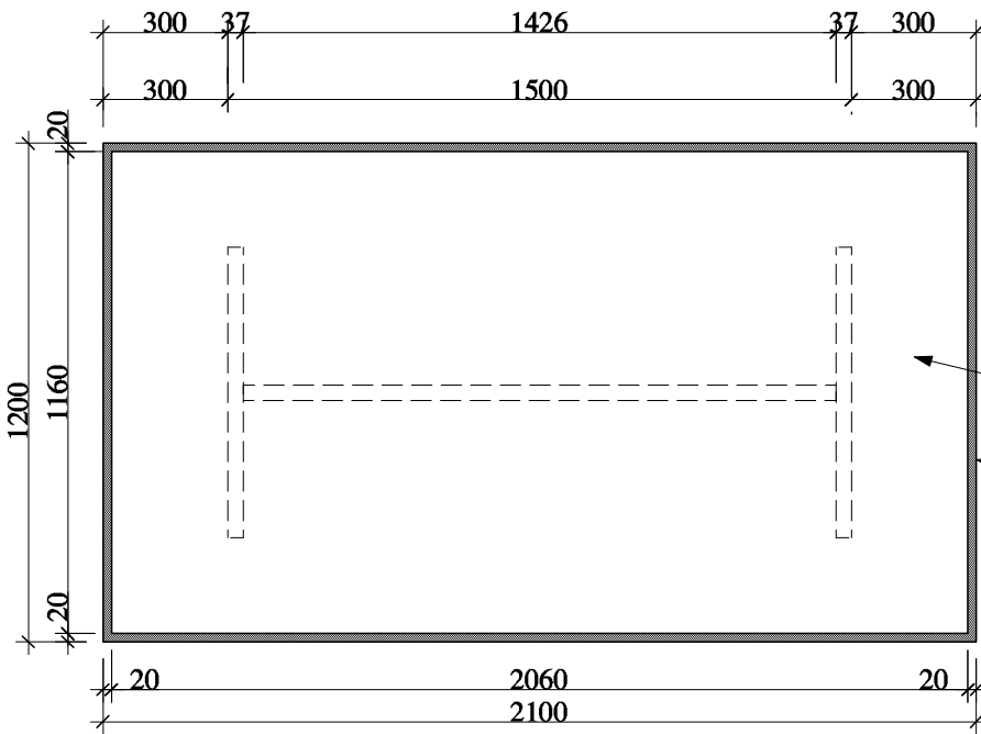
מבט על 1:20
