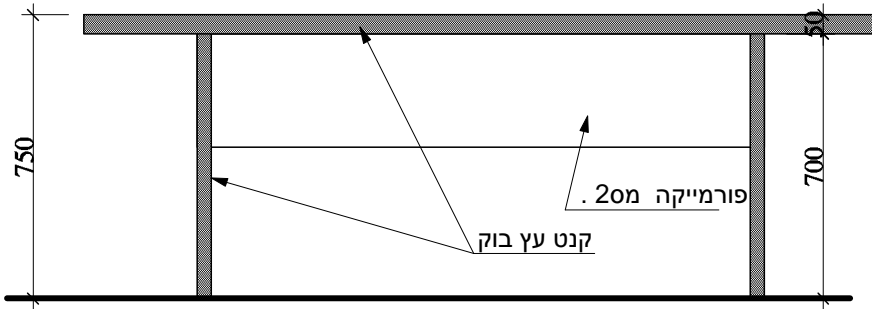
מבט חזיתי 1:20
