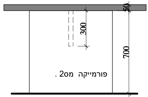
מבט צד 1:20
