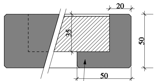
פרט חזית / מבט 1:2
