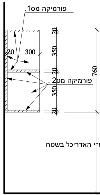
חתך רוחב 1:20
