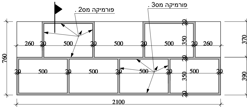
מבט חזיתי 1:20
