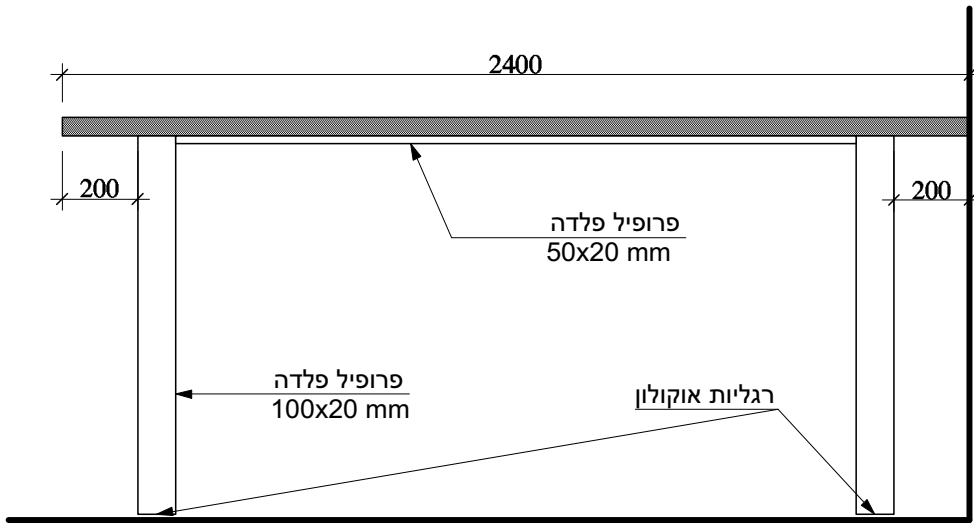
חזית 1:20
