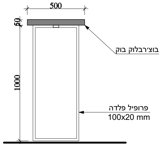
חתך 1:20
