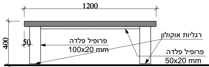
1:20 חזית
