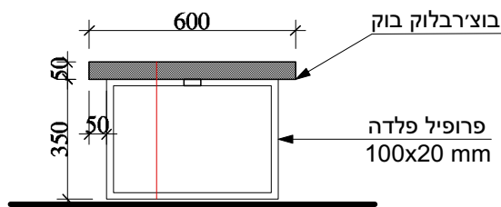
1:20 חתך
