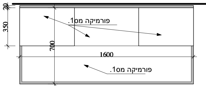
מבט על 1:20
