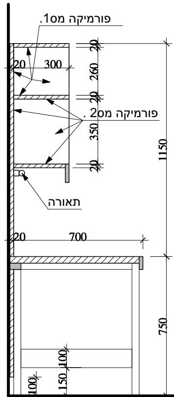
חתך רוחב 1:20
