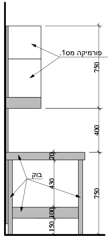
מבט צד 1:20
