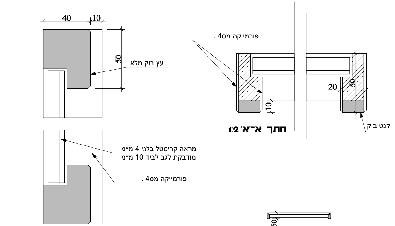
חתך א'א' 1:2
