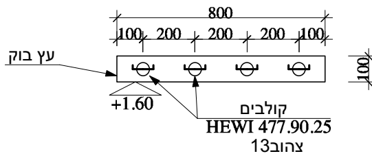
מבט חזית 1:20
