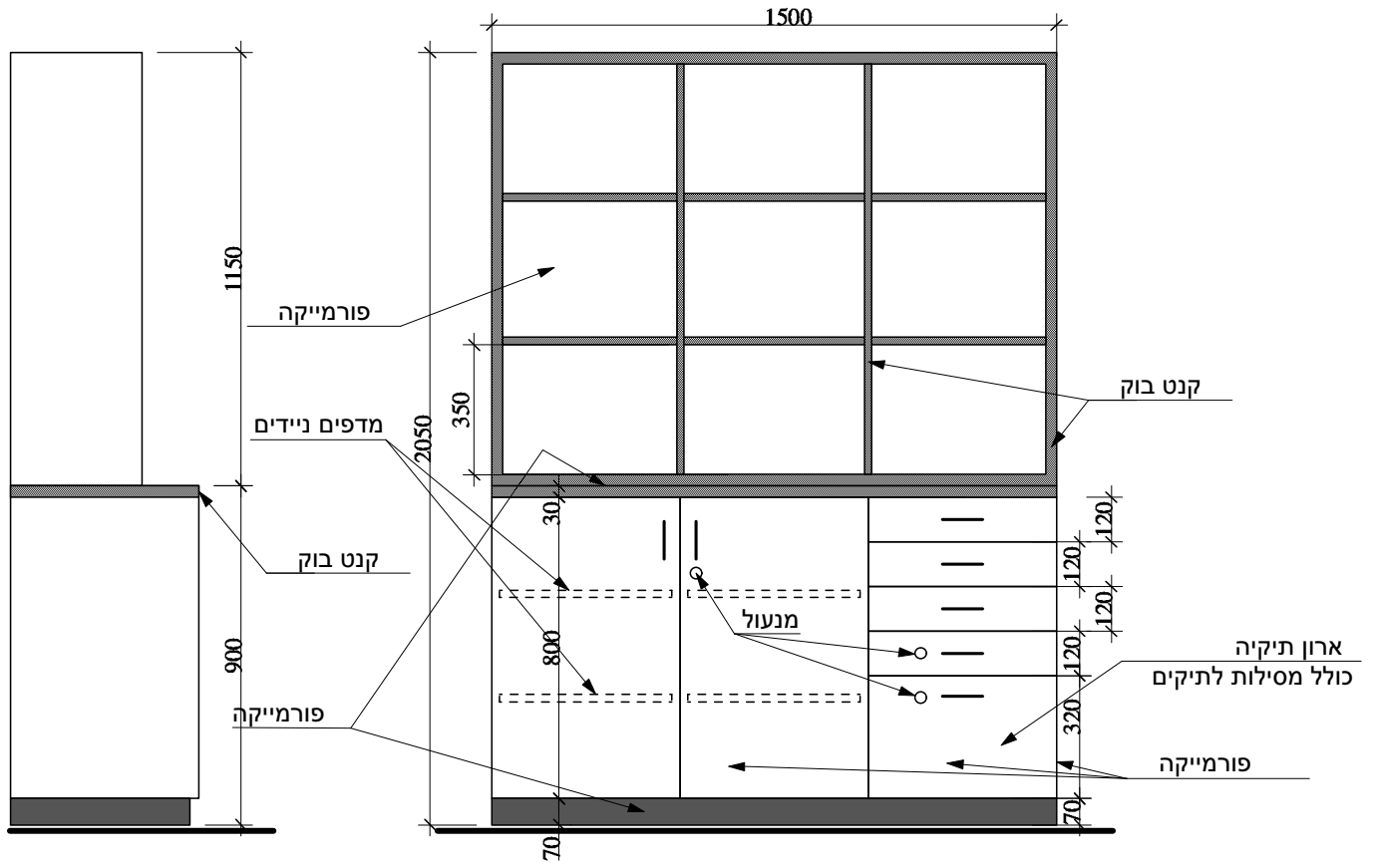
מבט צד 1:20
