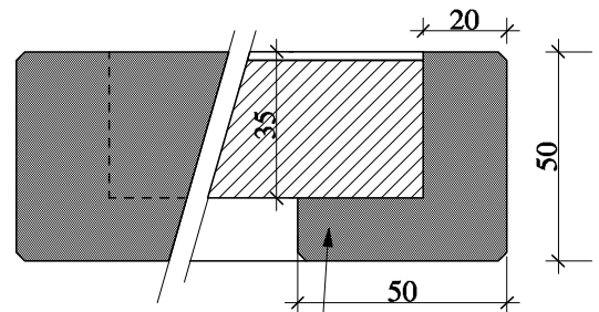
פרט חזית / מבט 1:2 עץ בוק
