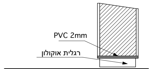
פרט חזית / מבט 1:2 עץ בוק
