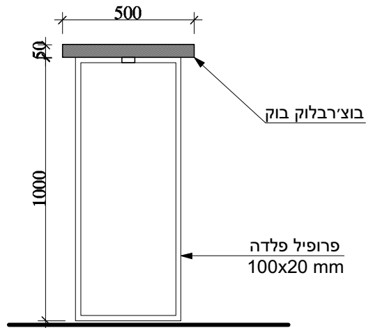
1:20 חתך
