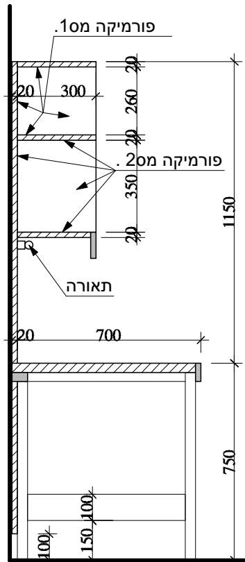
חתך רוחב 1:20
