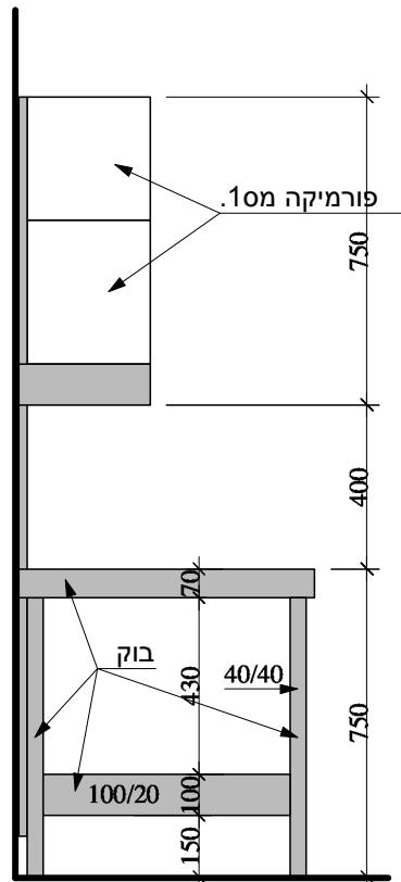
מבט צד 1:20
