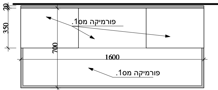
מבט על 1:20
