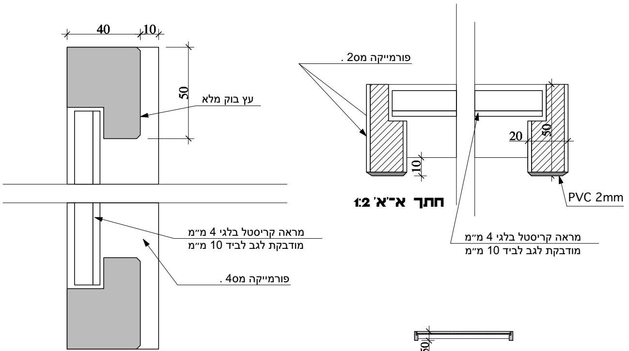
חתך א-א'
