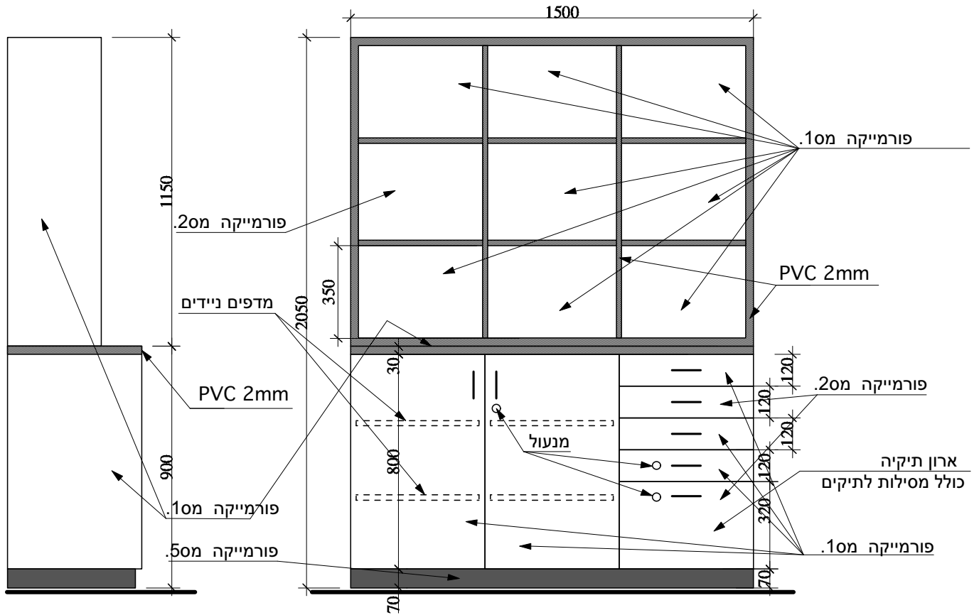
מבט צד 1:20
